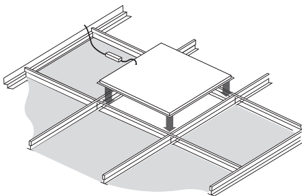
Рис. 1. Монтаж светильника в подвесной потолок типа «Армстронг» (модели PPL 595/R, PPL 595/U)
