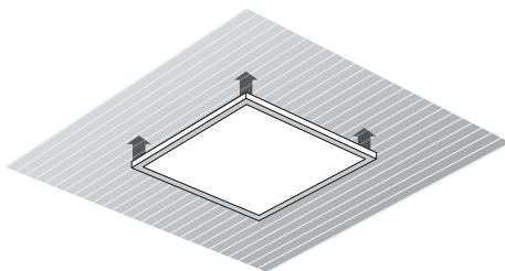
Рис. 2. Монтаж светильника накладным способом (модель PPL 595/U)
